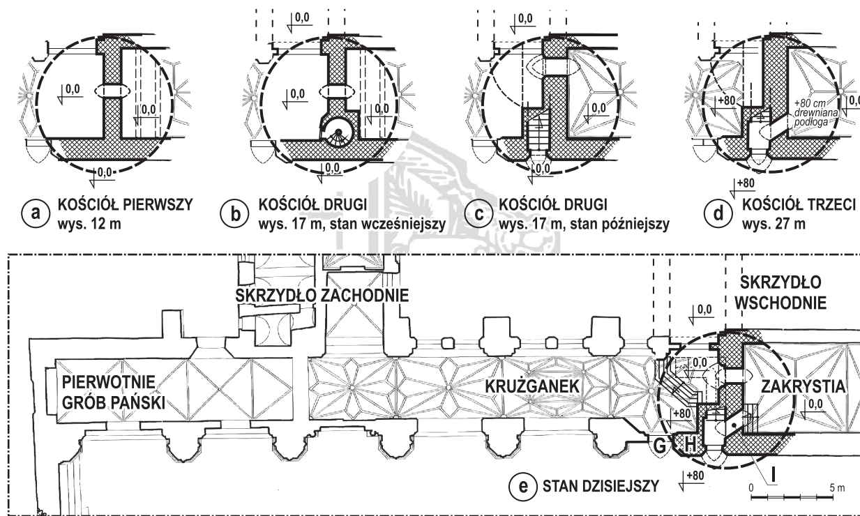
Il. 1. Kościół NMP w Toruniu, nawa północna, rzut w poziomie krużganek (inventaryzacja pomiarowa, wyk. Zbigniew Nawrocki, 1958)
