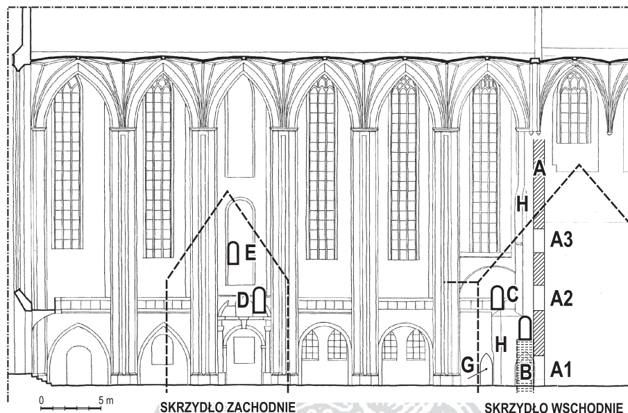
Il. 4. Kościół NMP w Toruniu, przekrój podłużny, widok w stronę nawy północnej; zaznaczono obszar styku muru północnego z budynkami klasztoru (inventaryzacja pomiarowa, wyk. Zbigniew Nawrocki, 1958)
