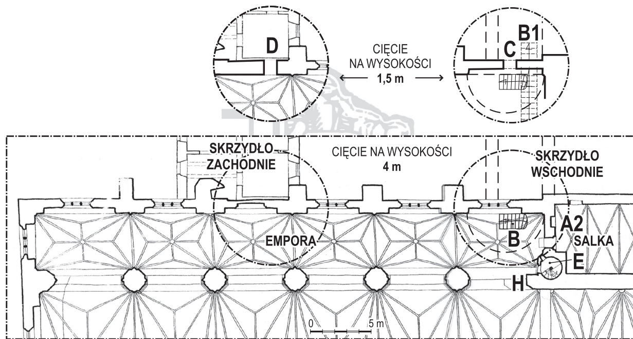
Il. 2. Kościół NMP w Toruniu, nawa północna, rzut w poziomie empory (inventaryzacja pomiarowa, wyk. Zbigniew Nawrocki, 1958)
