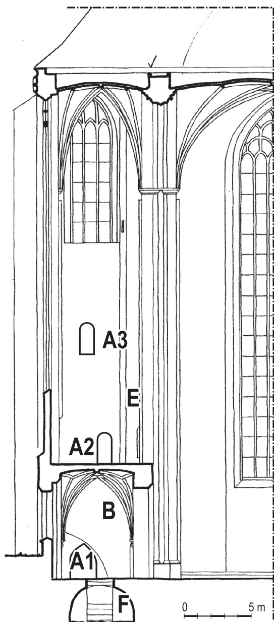
Il. 3. Kościół NMP w Toruniu, przekrój poprzeczny, widok na mur wschodni nawy północnej (inventaryzacja pomiarowa, wyk. Zbigniew Nawrocki, 1958)
